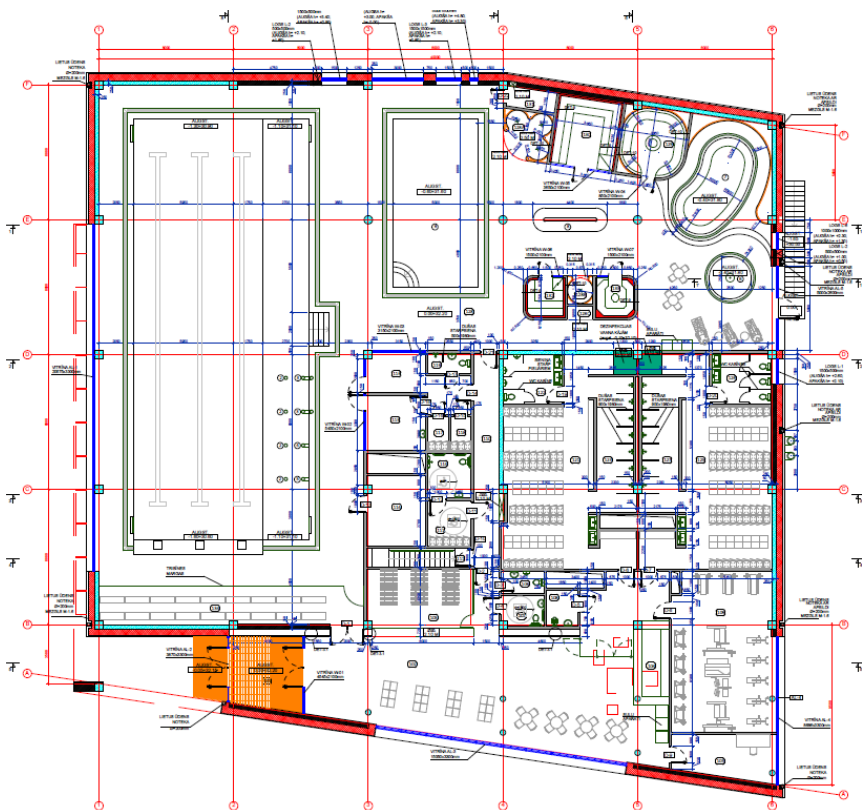
Attēls: 1.stāva plāns
